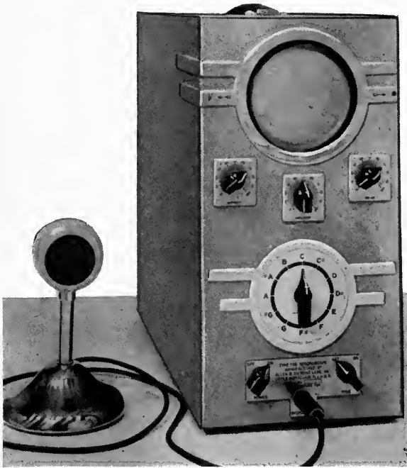
FIG. 4. The resonoscope.
